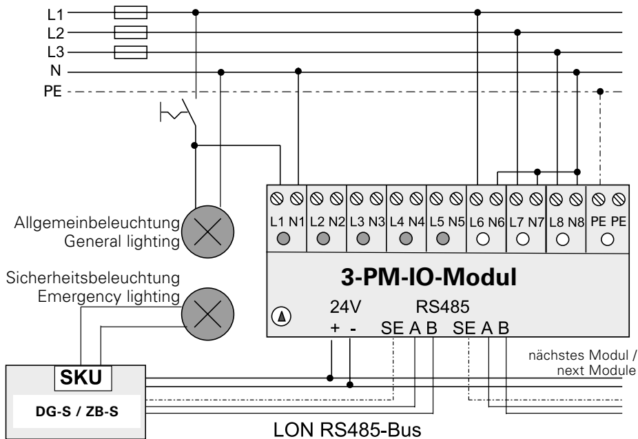
Bild 3 / fig. 3: Schaltung eines 3-PM-IO Moduls / Wiring of the 3-PM-IO module
