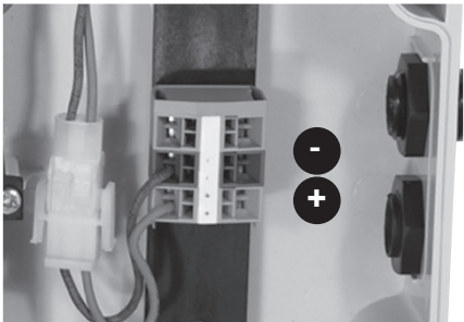
Bild 2a / fig. 2a / Fig. 2a Netzanschluss 24 V DC/Mains connec- tion 24 V DC/schéma des connexions 24 V CC
