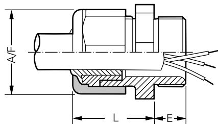
Cable gland
