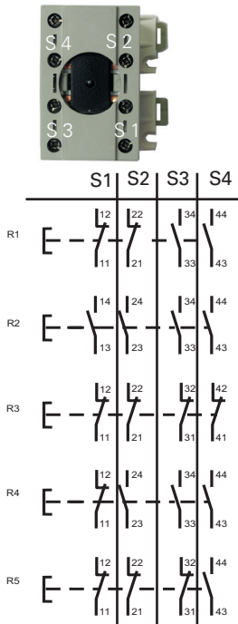
Drucktastersocket GHG41.11..R....; 1 x 4 polig
