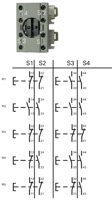
Drucktastersocket GHG41.11..R....; 2 x 2 polig
