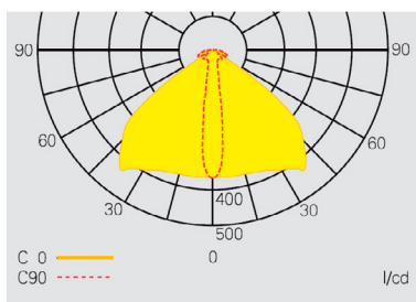
Kurva för ljusfördelning GuideLed SL 13032.2 CG-S utanpåliggande montering med asymmetrisk optik
