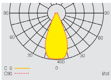
Kurva för ljusfördelning GuideLed SL 13042.2 CG-S utanpåliggande montering med symmetrisk optik
