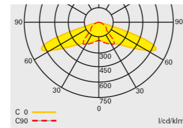
Ljusfördelningskurva 22011 LED CG-S med transparent kupa.
