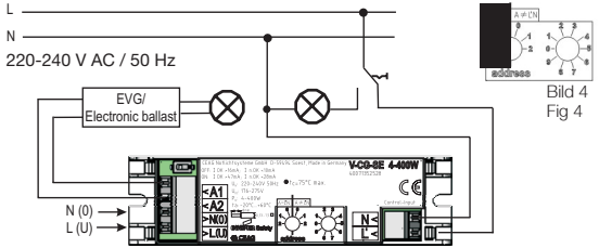
Bild 2 Anschluss an Stromkreise mit S+ oder STAR Technologie Fig 2 Connection to final circuits with S+ or STAR technology
