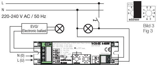
Bild 1 Anschluss an Stromkreise mit S+ oder STAR Technologie Fig 1 Connection to final circuits with S+ or STAR technology
