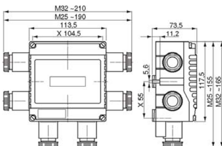
Boîtes de dérivation GHG 791 02
