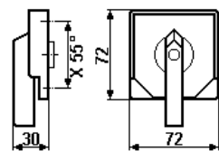
Steuerschalter Ex 29
