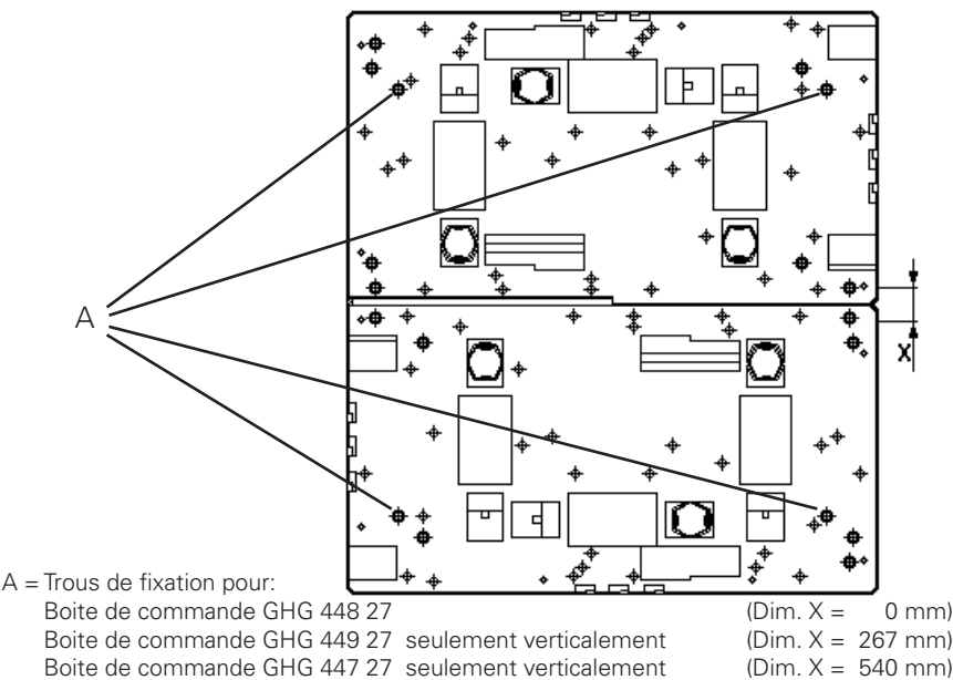
Fig. 8 Porte-appareils 2 x taille 3 pour fixation aux tubes, horizontalement
