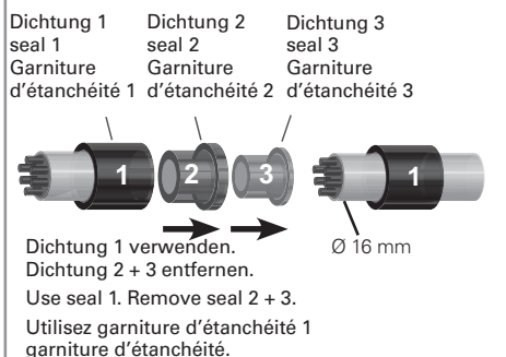
Fig. D Kabeldurchmesser Cable diameter Cable diameter z.B.: e.g.: e.g.: 16 mm; M25x1,5
