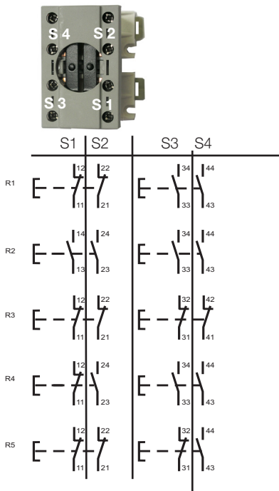
Kontaktbelegung
