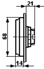
Doppeldrucktaster
