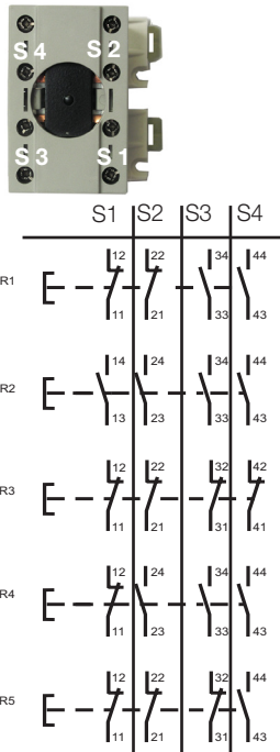
Drucktastersockel GHG41.11..R....; 2 x 2 polig
