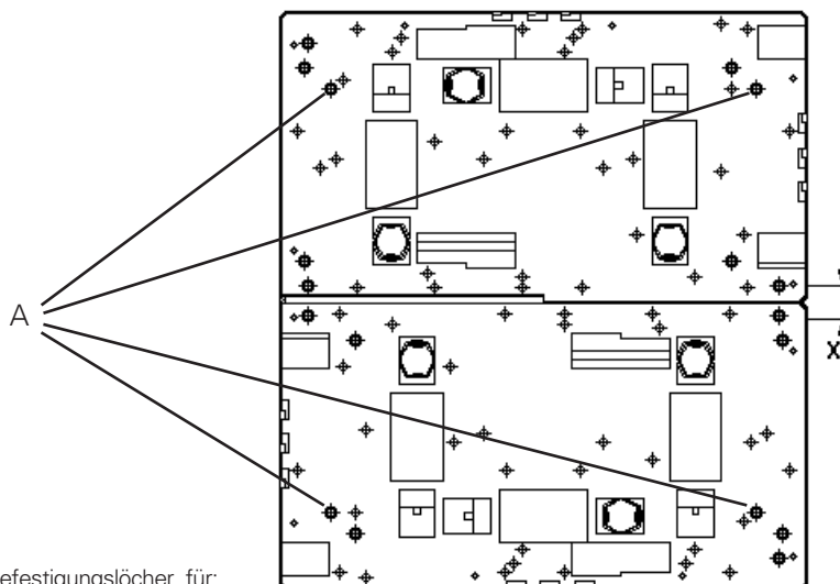
Bild 8 2 x Gerätehalter Größe 3 für Rohrbefestigung, horizontal
