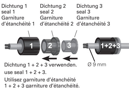
Fig. B Kabeldurchmesser Cable diameter Cable diameter z.B.: e.g.: e.g.: 9 mm; M25x1,5
