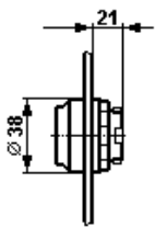
Drucktaster
