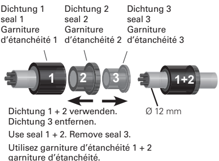
Fig. C Kabeldurchmesser Cable diameter Cable diameter z.B.: e.g.: e.g.: 12 mm; M25x1,5
