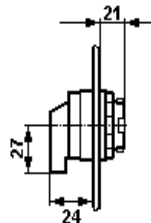
Steuerschalter
