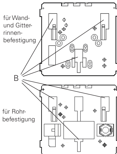
Gerätehalter Größe 1 für GHG 791 01
