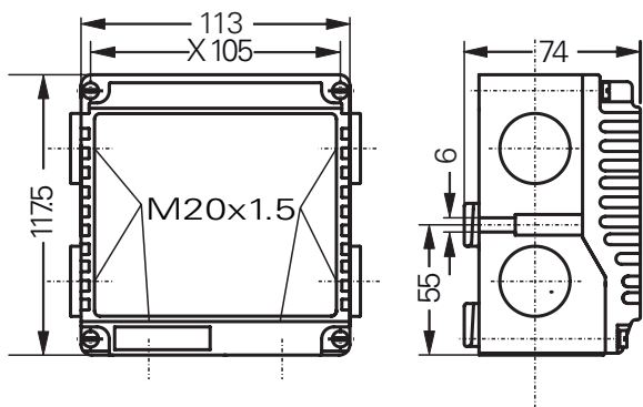
Terminal box GHG 791 02
