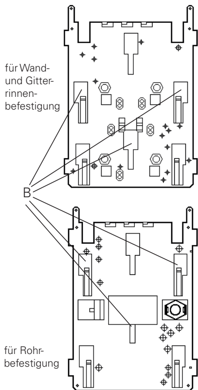
Gerätehalter Größe 2 für GHG 791 02
